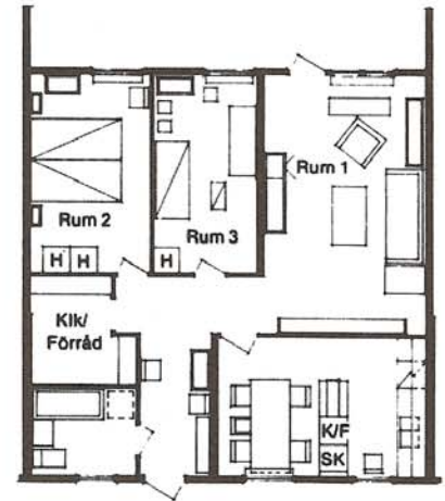
Figur 5. Plan av tidstypisk lägenhet från 1970-talet. Den visar tydligt den strikta funktionsuppdelningen och rumsliga separeringen av aktiviteter. (Bild ur Thiberg, 1985)
